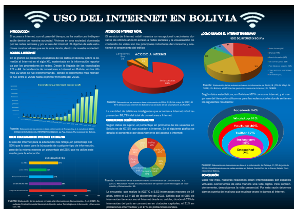
Categoría Gauss
