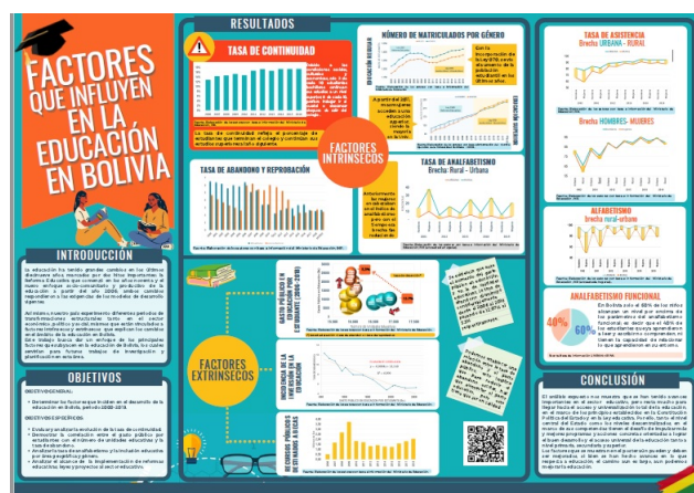
Categoría Gauss
